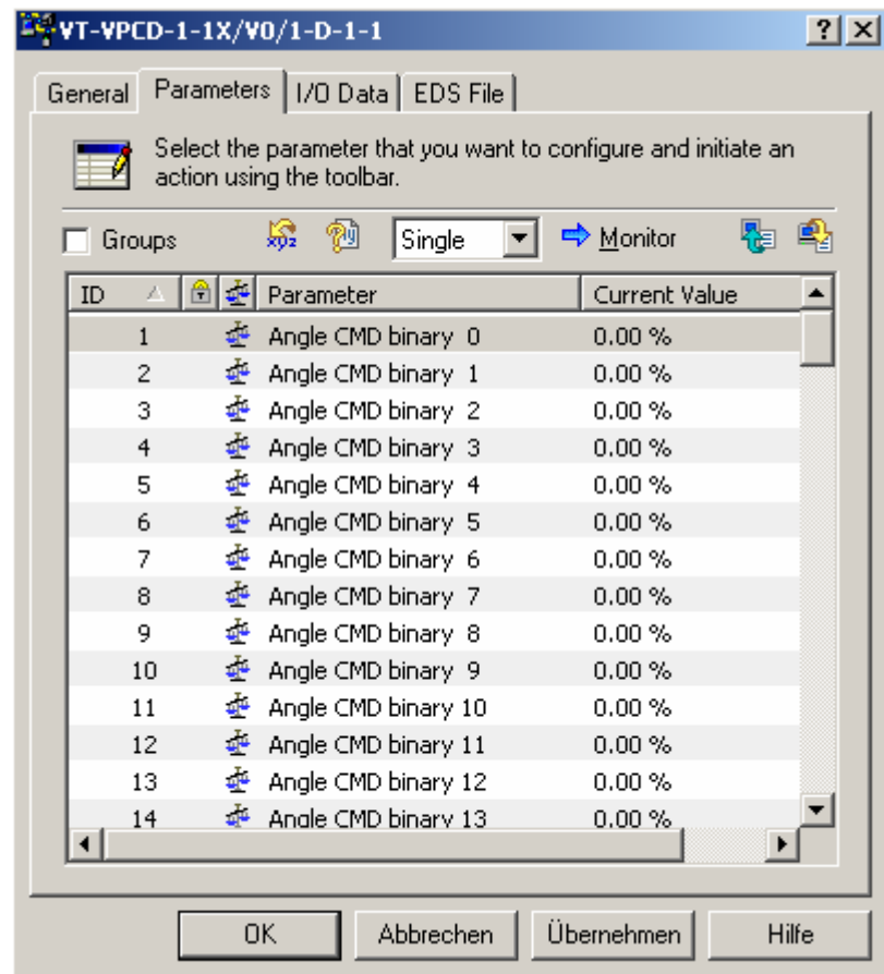
Fig. 7 : RSNetworx parameter screen .
